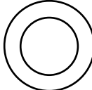
OD1/2, ID .319, L 1/4 Spacer
